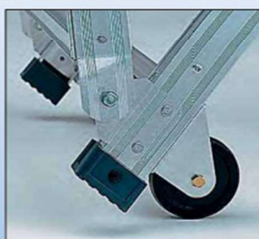
背面キャスター (φ 100)
